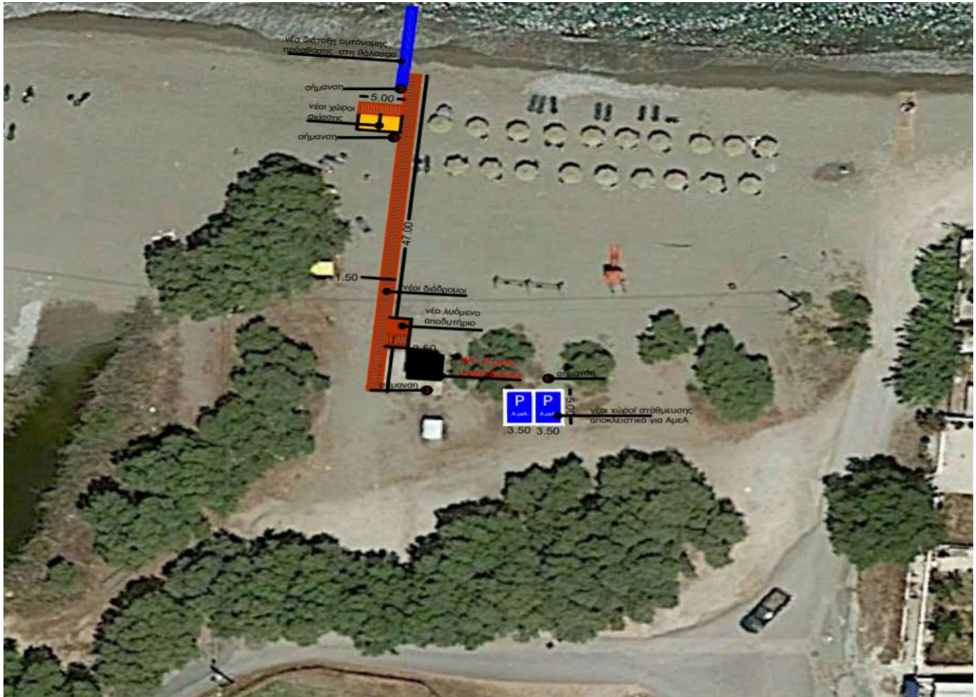
Εικόνα 4 Προτεινόμενη διάταξη για Α.μεΑ. στην παραλία Αγίου Παντελεήμονα
